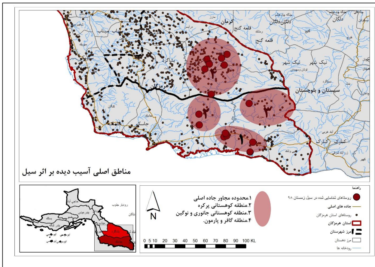
تصویر ۵۶- موقعیت مناطق اصلی آسیب دیده بر اثر سیل در استان هرمزگان
