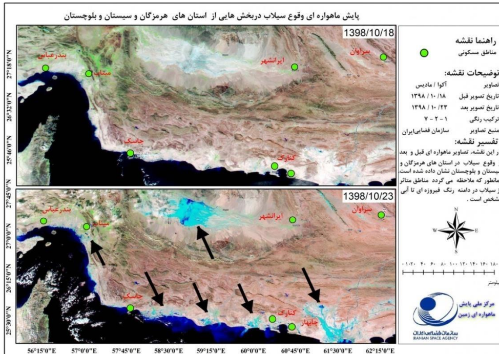
تصویر ۵- رواناب سطحی حاصل از سیلاب اخیر در بخش‌های مختلف جنوب استان سیستان و بلوچستان که بارنگ آبی فیروزه‌ای نشان داده شده است (منبع: سازمان فضایی ایران).
